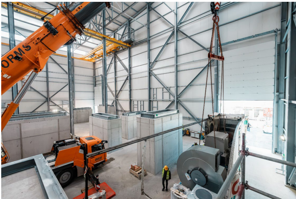
图片标题：将设备安装在预先准备好的混凝土基座上。
